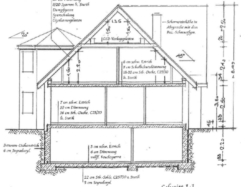
Schnitt 1-1
