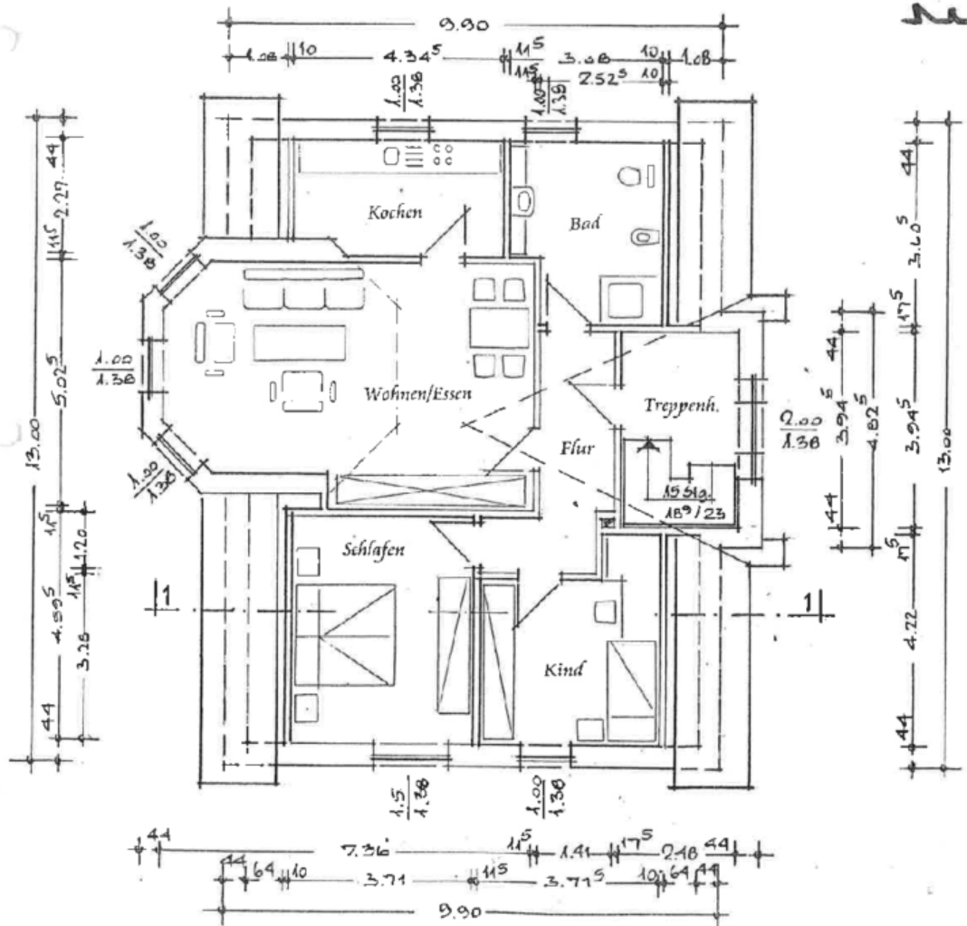
Dachgeschoss
